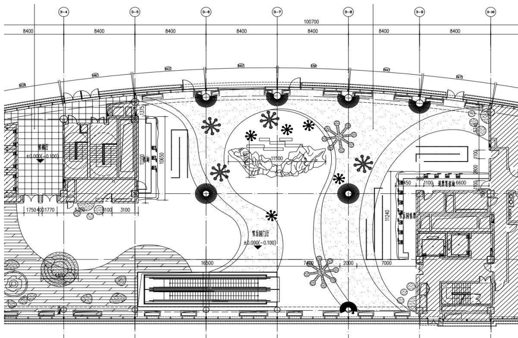
图 2.2 地面拼花示意图
