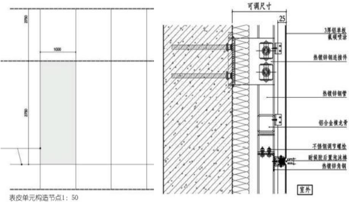
图 2.8 铝板幕墙立面、剖面示意图
