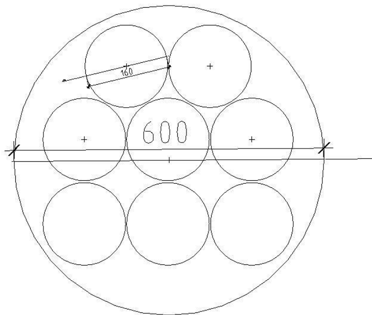
图 4.10 φ160*8 孔拖拉管断面图
